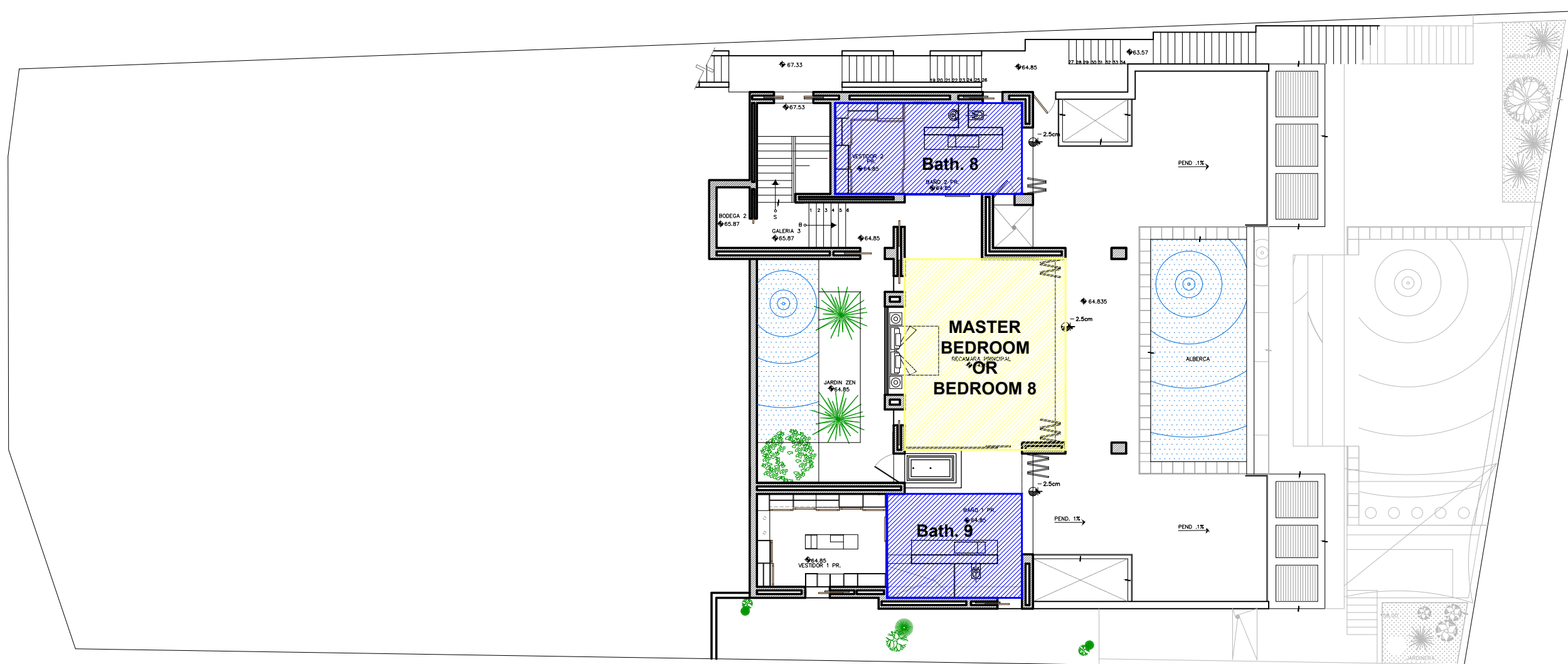
MANTEA CASA CABO-SECOND FLOOR
